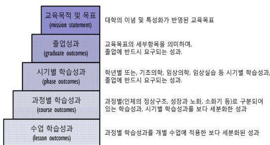
그림 1. 학습성과 체계도.
